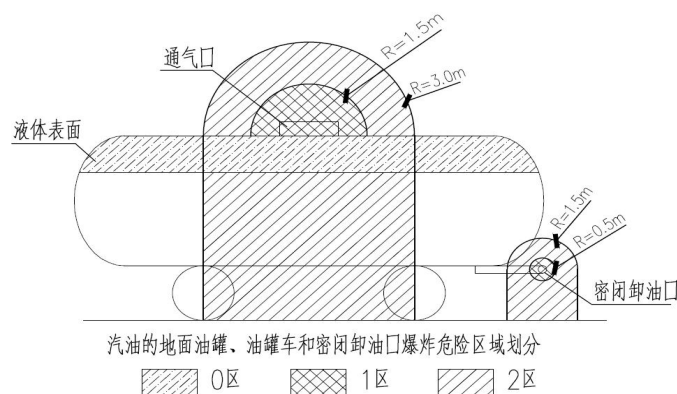
F3.3-2 汽油的油罐车和密闭卸油口的爆炸危险区域划分
