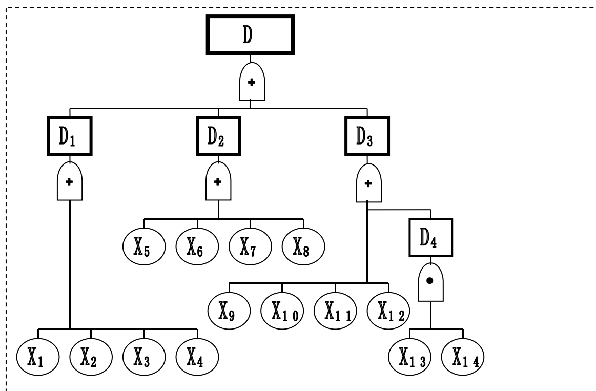
图 5.3-4 电气火灾事故树
