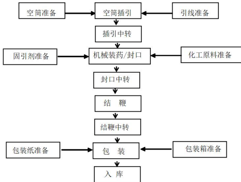
图 2-4-1 爆竹类生产流程图
