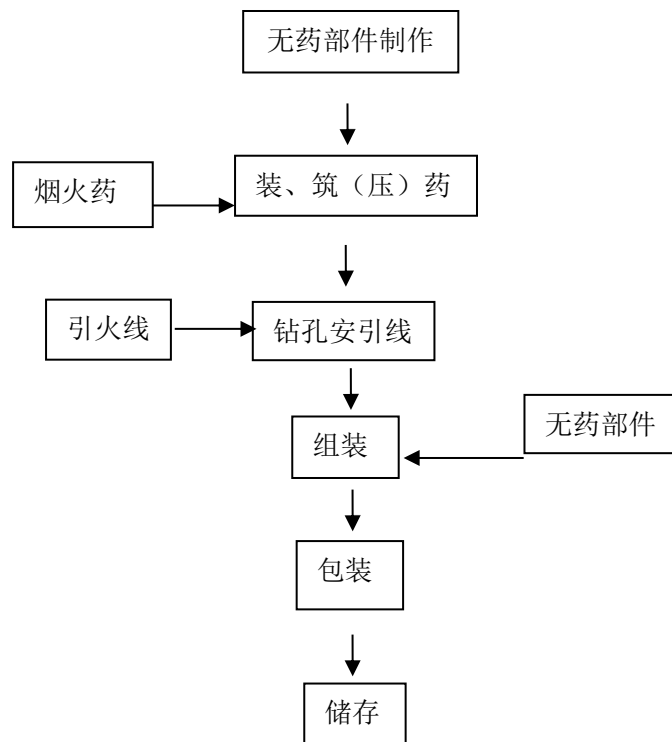
图 2-4-2 旋转类（无轴、有轴）生产工艺流程图
